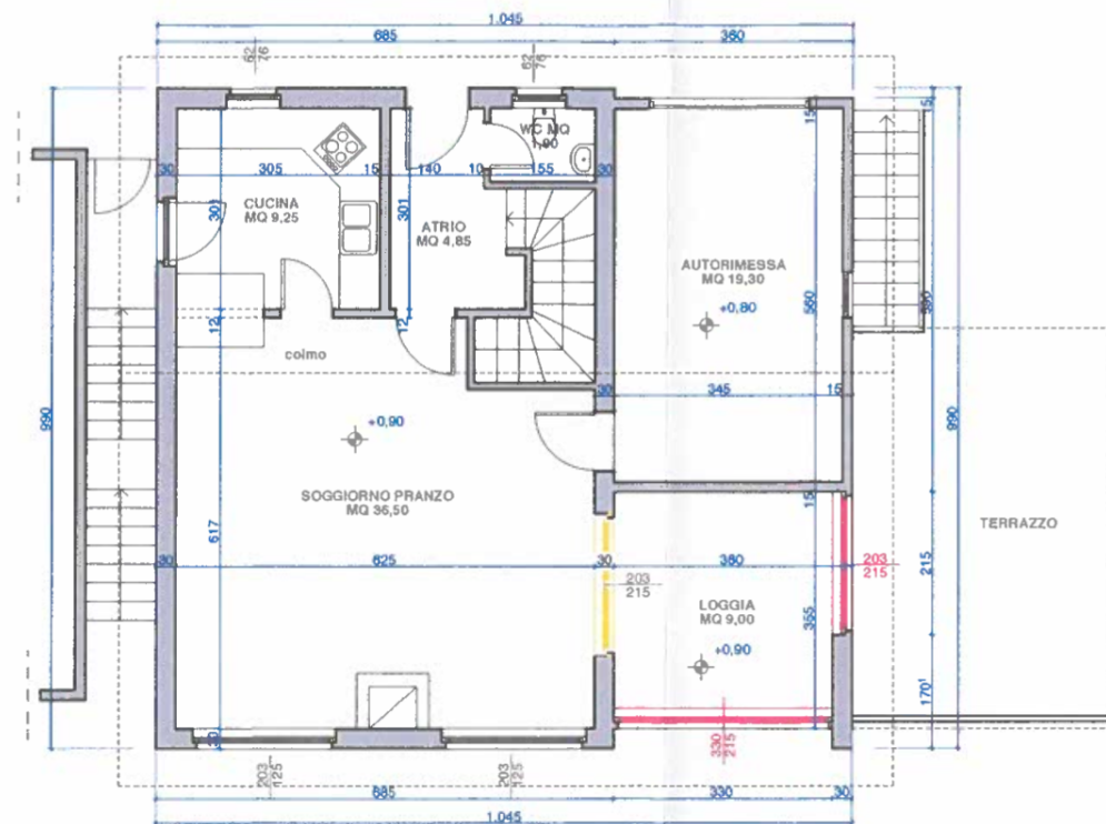
PIANTA PIANO TERRA progetto a posteriori
