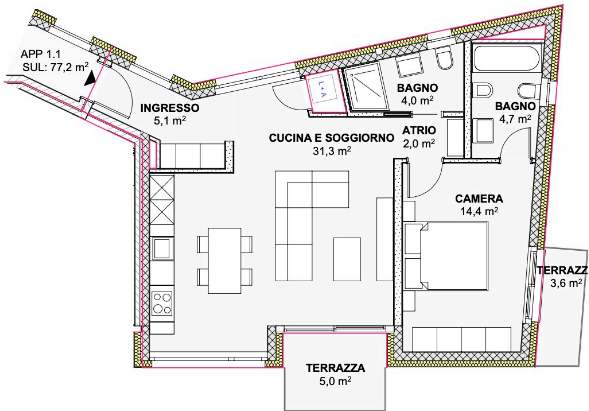
PIANTA
