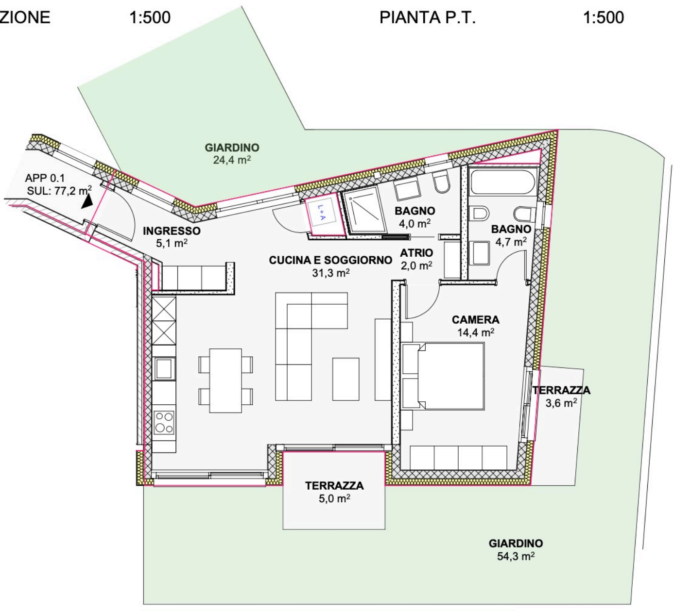
PIANTA 1:100
