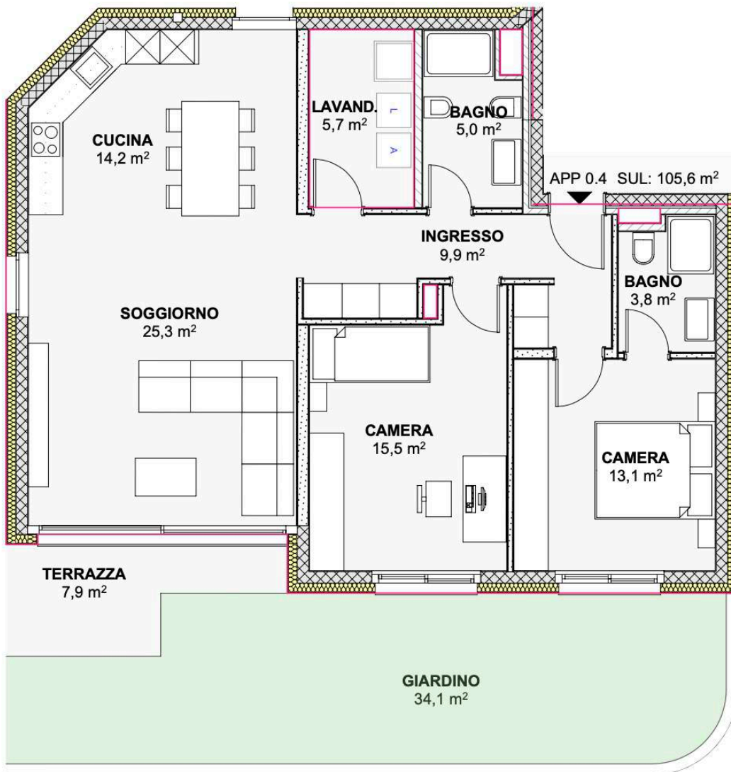
PIANTA
