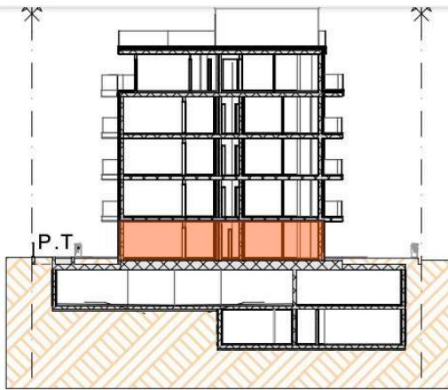
SEZIONE
